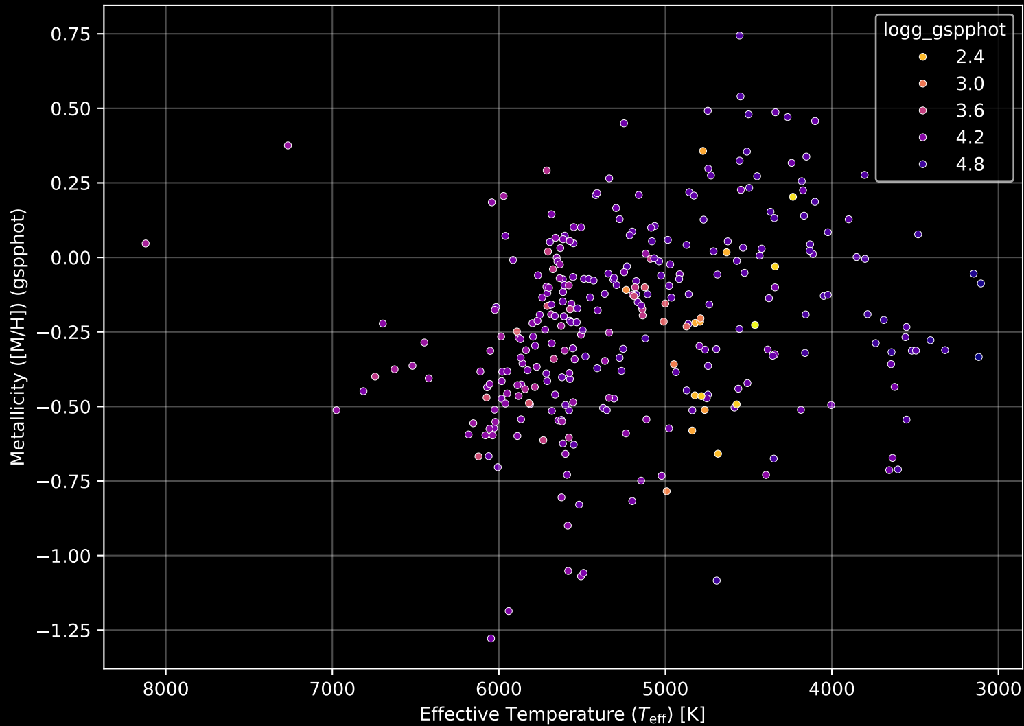
APOGEE DR17 Field: [179-57] Stellar Population Parameters (n= 314)
